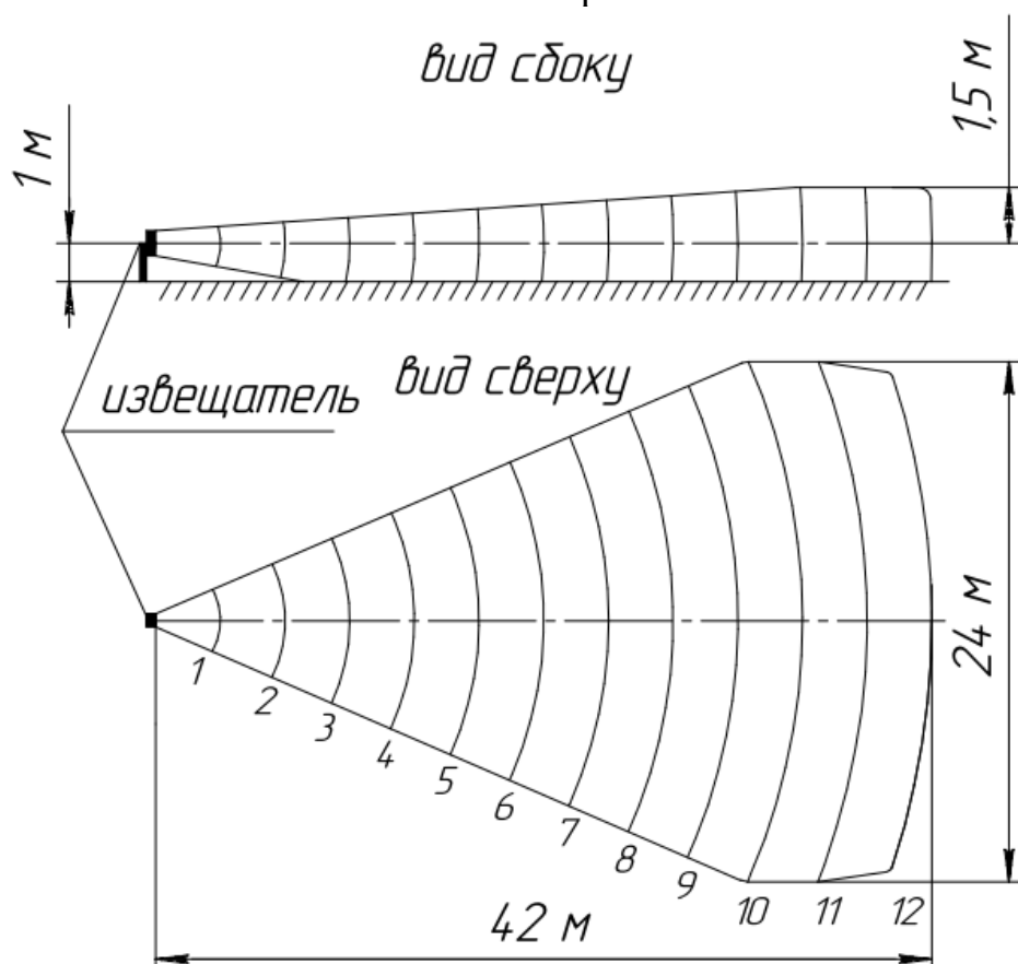
Рисунок 1.2 – Конфигурация зоны обнаружения, формируемой извещателем «ЗЕБРА-42(5,8)-В-Ethernet», установленными на опоре на высоте 1 м от поверхности земли
