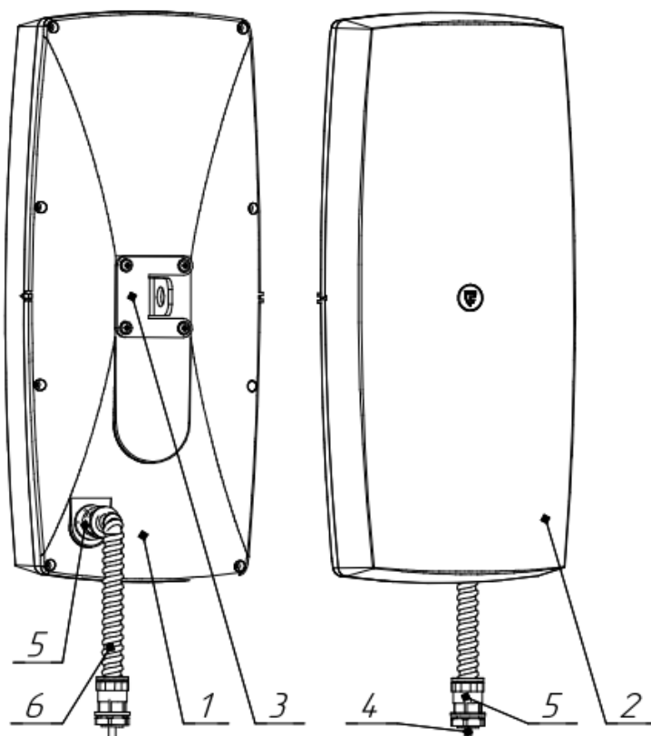
Рисунок 1.5 – Конструкция блока ПРМ-ПРД извещателя «ЗЕБРА-42(5,8)-III-Ethernet»
