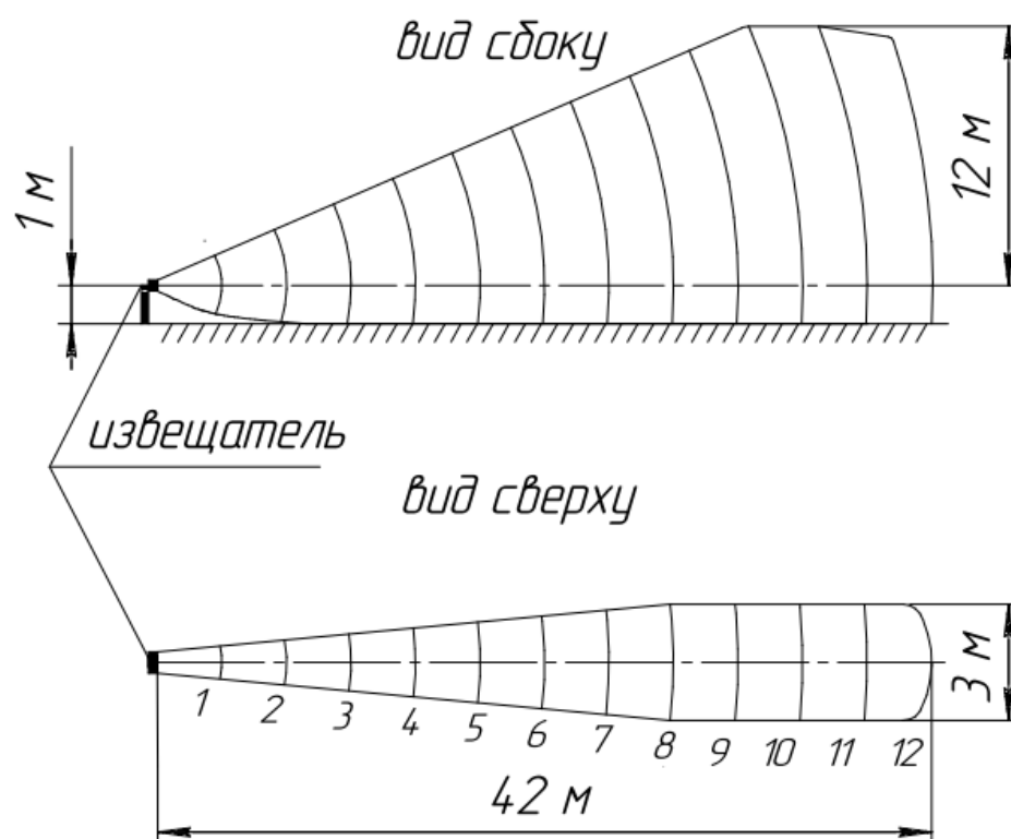
Рисунок 1.1 – Конфигурация зоны обнаружения, формируемой извещателем «ЗЕБРА-42(5,8)-Ш-Ethernet», установленными на опоре на высоте 1 м от поверхности земли
